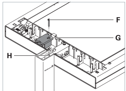
Fig. 3: Leuchtenkopf fixieren.
